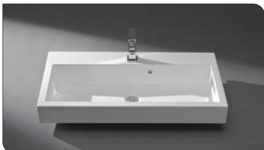
Einzelwaschtisch FARO mit Überlauf 612, 812, 1012 mm Becken mittig Weiß glänzend Beckeninnentiefe 128 mm Waschtischtiefe 460 mm
