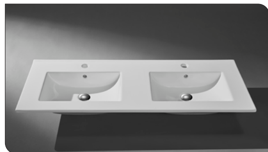
Doppelwaschtisch VERONA mit Überlauf 1210 mm Becken mittig / 2 Armaturlochbohrungen Weiß glänzend Beckeninnentiefe 160 mm Waschtischtiefe 460 mm
