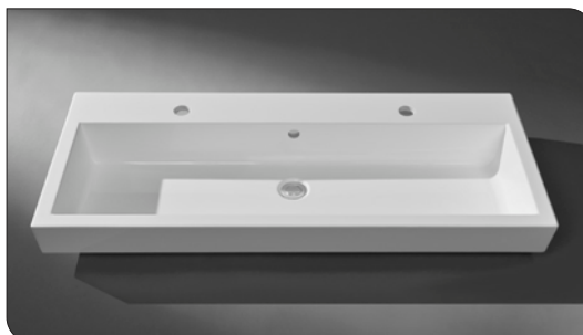
Doppelwaschtisch FARO mit Überlauf 1012 mm Becken mittig / 2 Armaturlochbohrungen Weiß glänzend Beckeninnentiefe 128 mm Waschtischtiefe 460 mm
