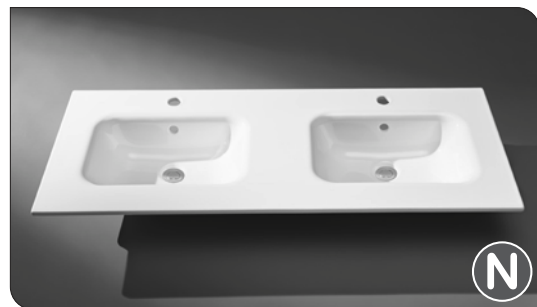
Doppelwaschtisch NORDIC mit Überlauf 1210 mm Becken mittig / 2 Armaturlochbohrungen Weiß glänzend Beckeninnentiefe 120 mm Waschtischtiefe 460 mm
