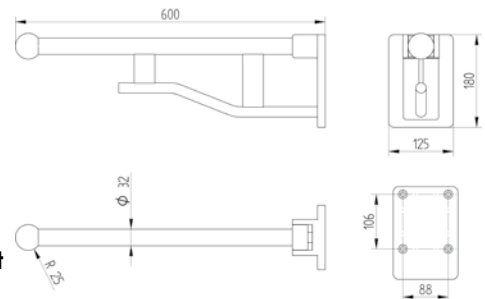
900 4710 010 Stützklappgriff 600 mm nach oben klappbar, gebremste Ausführung, Oberseite des Griffs mit Kunststoff ummantelt. Das Befestigungs-Set bitte separat bestellen. Siehe Seite 145 foldable grab rail 600 mm
