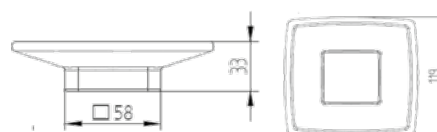
900 1552 905 Seifenschale für Multifunktionshalter mit Kunststoffring soap dish for multifunctional holder
