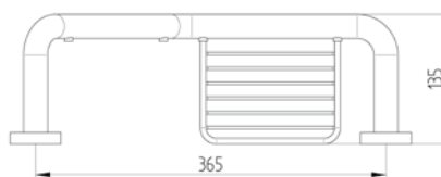
900 3031 010 Wannengriff 135° abgewinkelt mit Korb links wie rechts montierbar angled bath grab bar with basket
