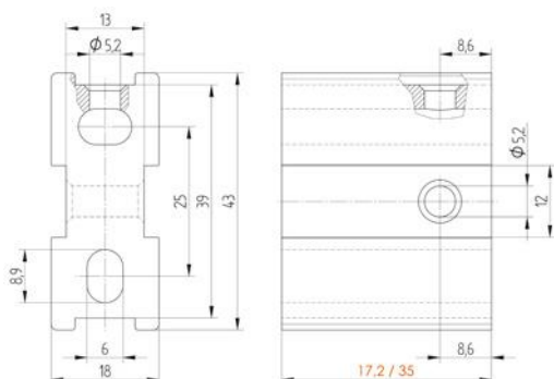
900 9004 000 Wandbefestiger kurz 17,2 mm zu 900 4730 + 4745 + 4760 + 4775 + 4776 + 4780 + 4796 alle Konsolen, 900 4797 + 4798 obere Konsolen wall mounting set
