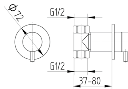
280 6540 010 Wandeinbauventil für Warmwasser mit Unterputz-Einbaukörper 1/2" linksschließend
