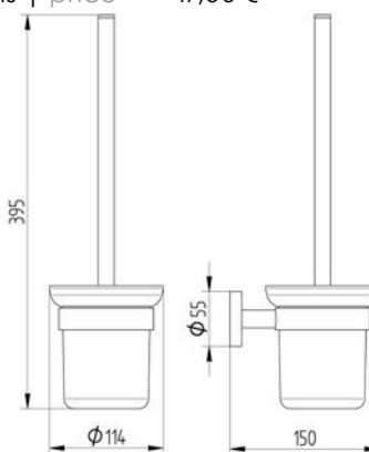
190 2200 015 Toilettenbürstengarnitur mit Schallschutzring passender WC-Ersatzbürstenkopf weiß, Ø 73 mm, Art.-Nr. 100 2573 030 toilet brush set
