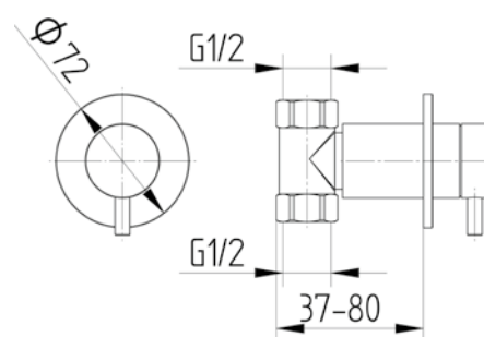
280 6541 010 Wandeinbauventil für Kaltwasser mit Unterputz-Einbaukörper 1/2" rechtsschließend
