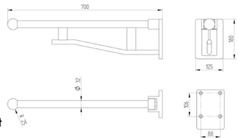
900 4711 010 Stützklappgriff 700 mm nach oben klappbar, gebremste Ausführung, Oberseite des Griffs mit Kunststoff ummantelt. Das Befestigungs-Set bitte separat bestellen. Siehe Seite 145 foldable grab rail 700 mm
