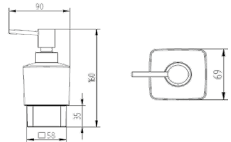
900 1553 905 Seifenspender für Multifunktionshalter Füllmenge 270 ml soap dispenser for multifunctional holder
