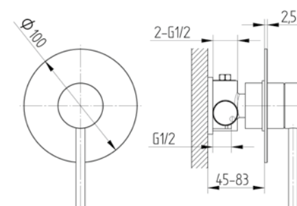
280 6250 010 Brause-Einhebelmischbatterie mit Unterputz-Einbaukörper 1/2" mit Keramik-Kartusche Verlängerungs-Set s. Ersatzteile single lever shower mixer
