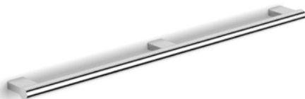
900 4780 010 Haltegriff 800 mm mit 3 Konsolen, Rohr ø 32 mm grab handle 800 mm
