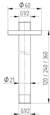
900 6955 010 | 900 6955 040 black Brausearm für Deckenmontage 120 mm, 1/2"
