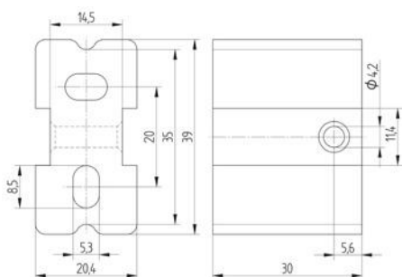
100 9011 000 Wandbefestiger zu 480 3030
