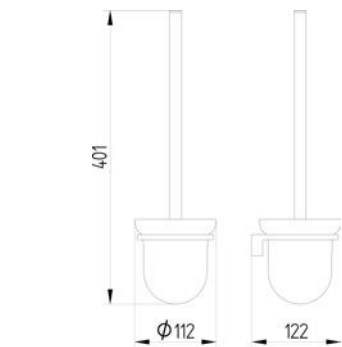
360 2200 010 Toilettenbürstengarnitur passender WC-Ersatzbürstenkopf weiß, Ø 77 mm, Art.-Nr. 100 2577 030 toilet brush set
