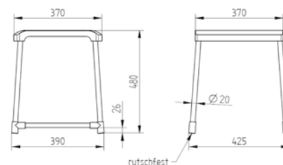
900 4721 010 Bad-/Dusch-Hocker mit weißer Sitz- fläche bathroom stool with white seat
