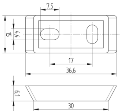
100 9010 000 Wandbefestiger zu 480 1410 + 1415 + 2100
