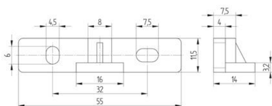
100 9009 000 Wandbefestiger zu 480 1500 + 2000 + 2010
