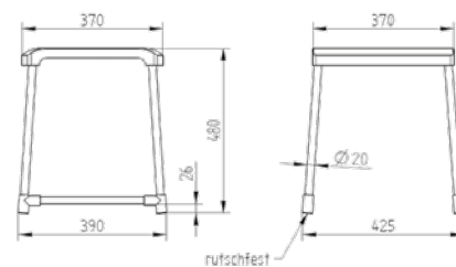
900 4720 010 Bad-/Dusch-Hocker mit schwarzer Sitzfläche bathroom stool with black seat
