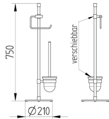
910 4505 010 Design-Ständer WC mit Glasfuß passender WC-Ersatzbürstenkopf schwarz, Ø 77 mm, Art.-Nr.100 2577 040 free standing pole WC
