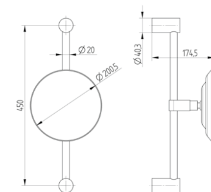
950 5125 010 Kosmetikspiegel – Wandmodell unbeleuchtet, 5-fach Ø 200 mm, höhenverstellbar cosmetic mirror - wall-mounted
