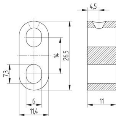
100 9008 000 Wandbefestiger zu 480 1600
