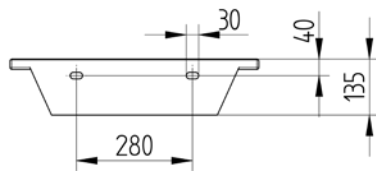
902 8060 030 Waschtisch aus Mineralguß 600 mm mit Überlauf
