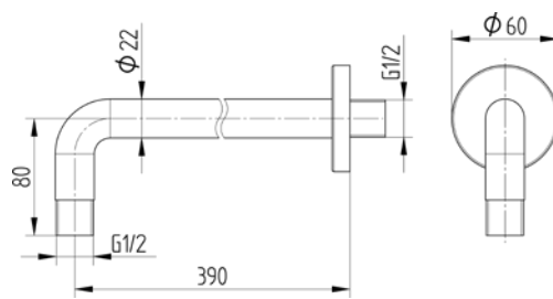
900 6944 010 NEU Brausearm für Wandmontage 390 mm, 1/2" extra stabile Ausführung shower arm wall-mounted
