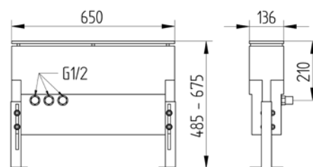
900 7605 010 Montagegestell mit Montageplatte für alle Wannenrandarmaturen mit Wasserauffangbehälter, 3 Anschlüsse (Kalt, Warm, Abgang), Montagematerial inkl. Ablauf- schlauch mounting frame with mounting plate
