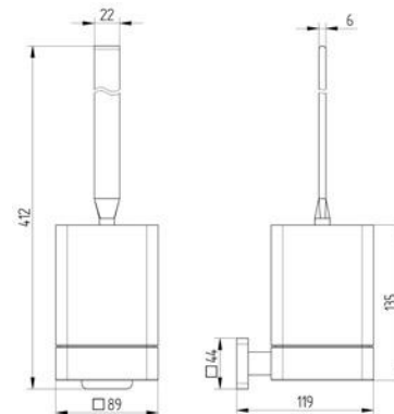
240 2200 010 Toilettenbürstengarnitur mit Schallschutzing passender WC-Ersatzbürstenkopf weiß, Ø 75 mm, Art.-Nr. 100 2575 030 toilet brush set
