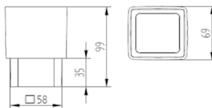
900 1551 905 Mundspülglas für Multifunktionshalter mit Kunststoffring glass for multifunctional holder
