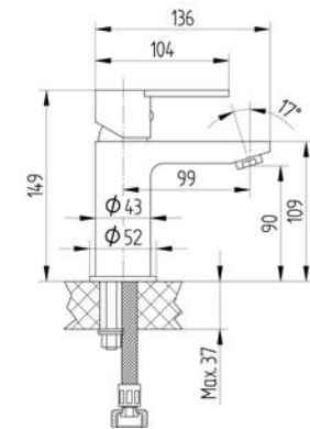
180 6002 010 Waschtisch-Einhebelmischbatterie mit Keramik-Kartusche mit Flexschläuchen 3/8" single lever basin mixer
