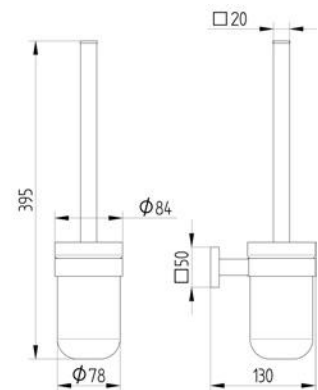
420 2200 040 Toilettenbürstengarnitur mit Schallschutzring passender WC-Ersatzbürstenkopf schwarz, Ø 69 mm, Art.-Nr. 100 2569 040 toilet brush set
