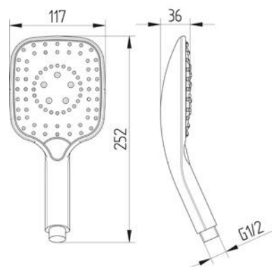
900 7362 040 Handbrause black 3-fach verstellbar mit Umstellung per Druckknopf Kunststoff
