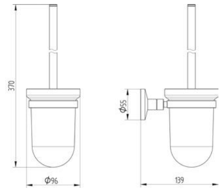
170 2200 010 Toilettenbürstengarnitur passender WC-Ersatzbürstenkopf weiß, Ø 67 mm, Art.-Nr. 100 2567 030 toilet brush set
