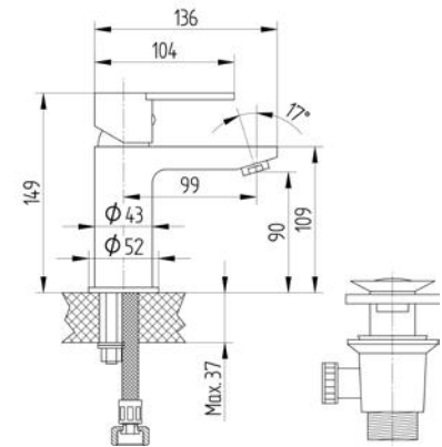
180 6000 010 Waschtisch-Einhebelmischbatterie mit Keramik-Kartusche mit Ablaufgarnitur 1 1/4" mit Flexschläuchen 3/8" single lever basin mixer
