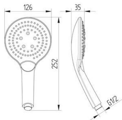
900 7361 040 Handbrause black 3-fach verstellbar mit Umstellung per Druckknopf Kunststoff
