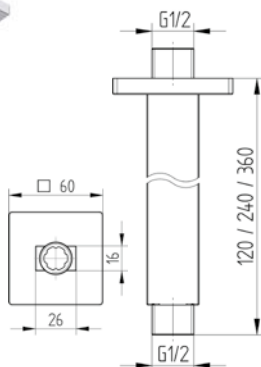
900 6962 010 Brausearm für Deckenmontage 120 mm, 1/2"
