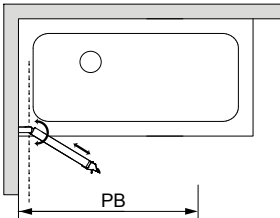
Draufsicht Einbausituation
