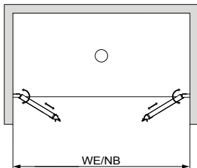
Draufsicht Einbausituation
