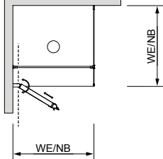
Draufsicht Einbausituation
