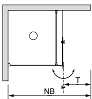
Draufsicht Einbausituation
