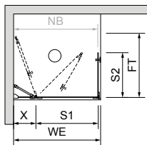
Draufsicht Einbausituation
