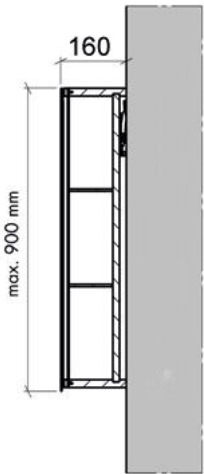
MIRR 6 AUFBAU | for installation on the wall
